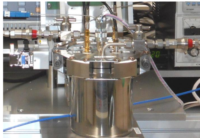
300°C対応測定用試作治具外観図
